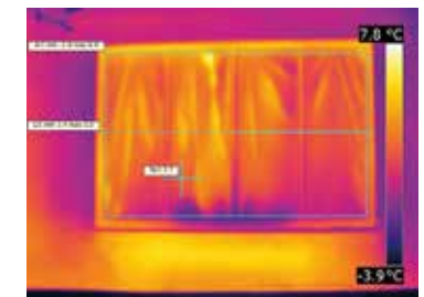
Außenaufnahme Thermografie-/Infrarotbild eines Fensters, Vorhang geschlossen
