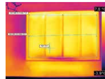
Außenaufnahme Thermografie-/Infrarotbild eines Fensters, Vorhang geöffnet
